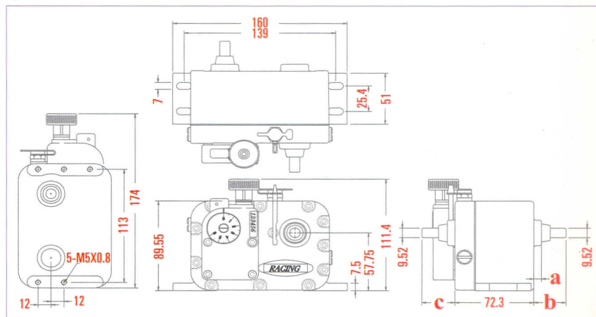
尺寸圖 Specification
